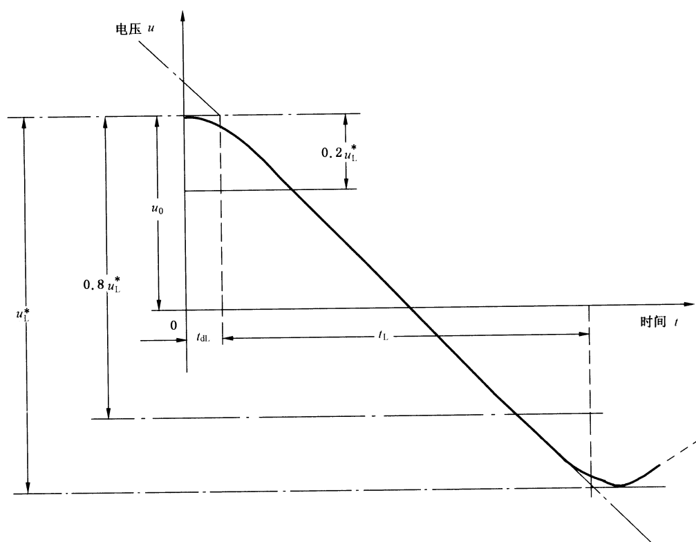
图 16 有时延的线路侧瞬态电压以及圆形的波峰导出 u_L^* 、 t_L 和 t_{dl} 方法的说明
