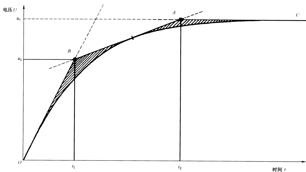
图 E.3 用四参数表示回路的预期瞬态恢复电压——E.2 c) 3) i) 的情况
