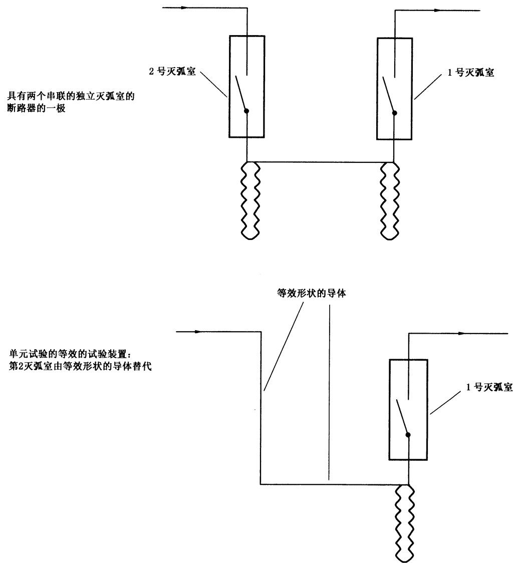
图 24 多于一个独立灭弧室的断路器的单元试验的等效试验装置
