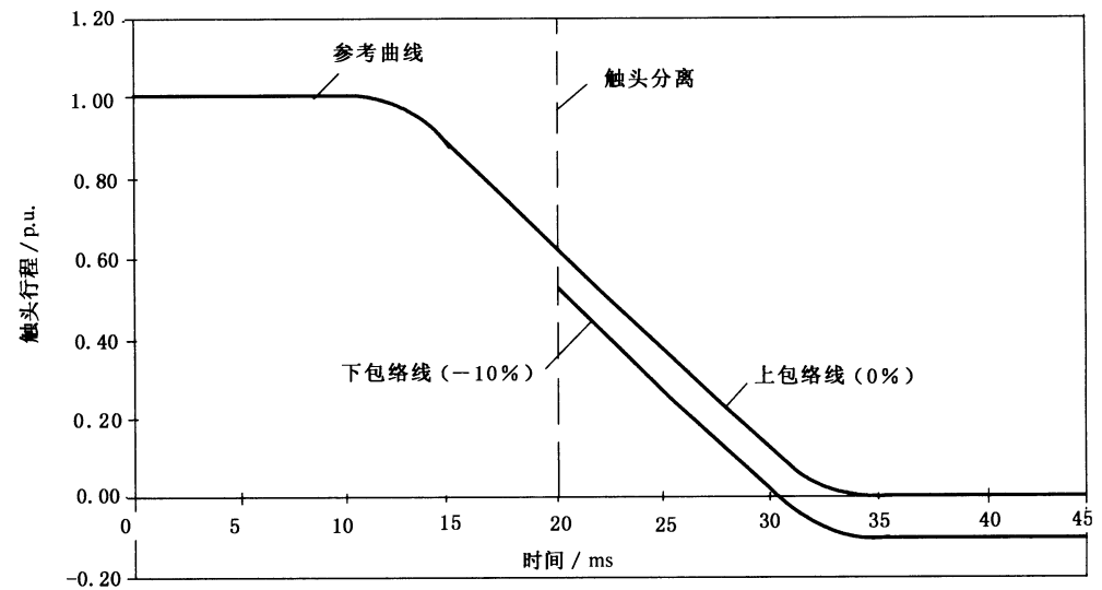
d) 具有以参考曲线为基准完全下移的规定的包络线(0%,-10%)的参考机械行程特性(理想曲线), 本例中触头分离时刻为 t = 20\text{ ms}
