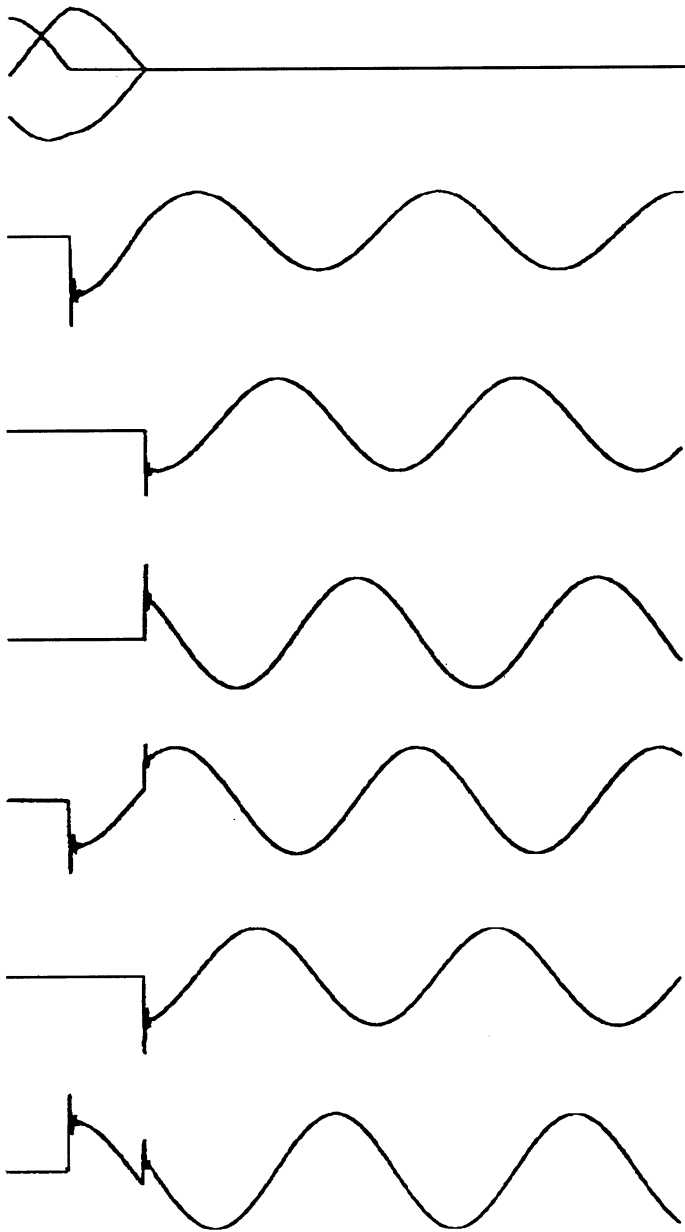
图 O.2 如图 25a)所示的,表明三相开断过程中对称电流、相对地和相间电压的波形示例
