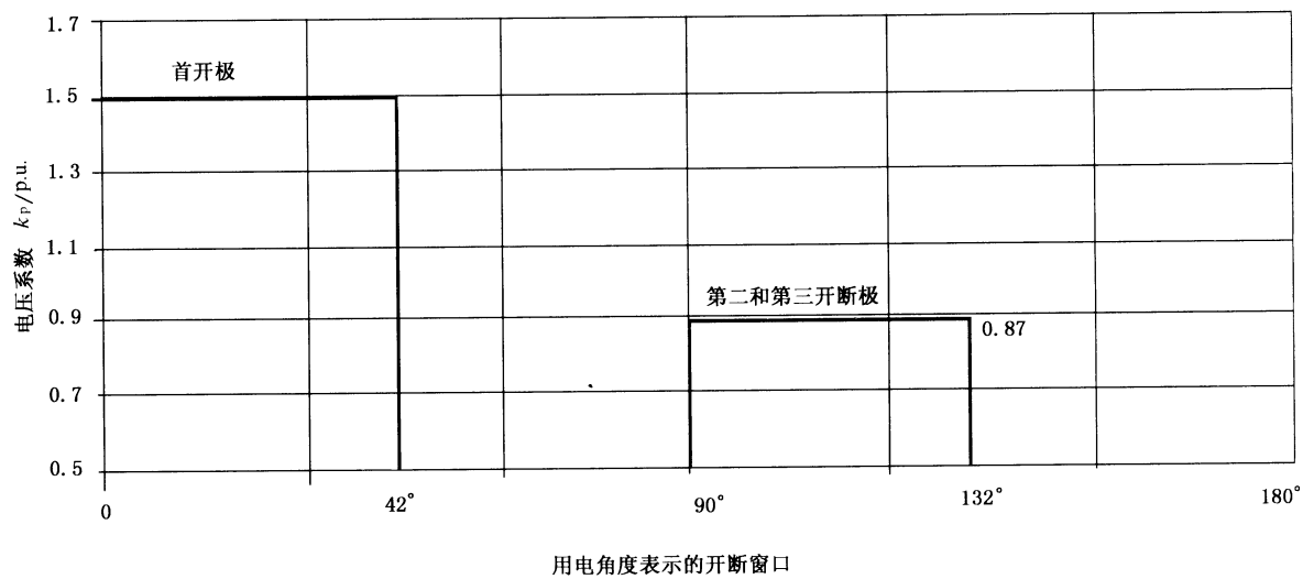
图 38 对于首开极系数为 1.5 的系统,决定各极 TRV 的开断窗口和电压系数 k_p 的图形表示
