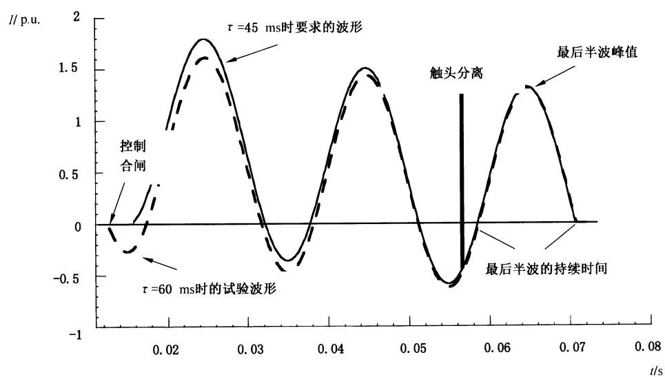
大半波后电流零点开断
