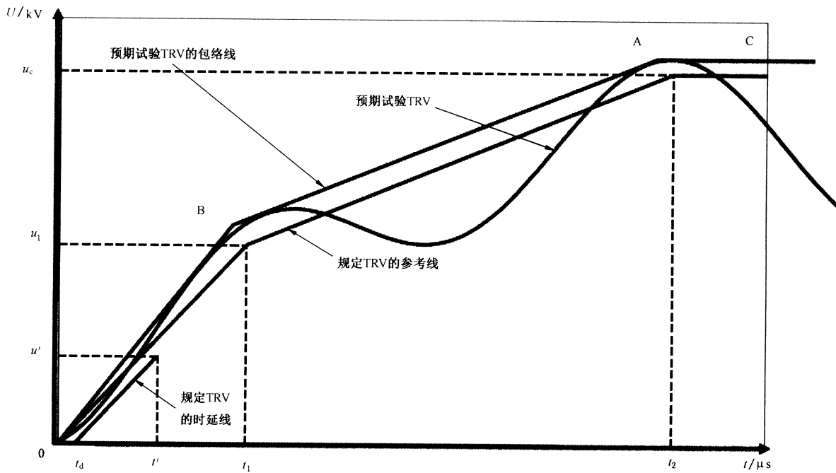
图 39 满足型式试验条件的、用四参数包络线表示的预期试验的 TRV 示例： 具有四参数参考线的规定的 TRV 的情况
