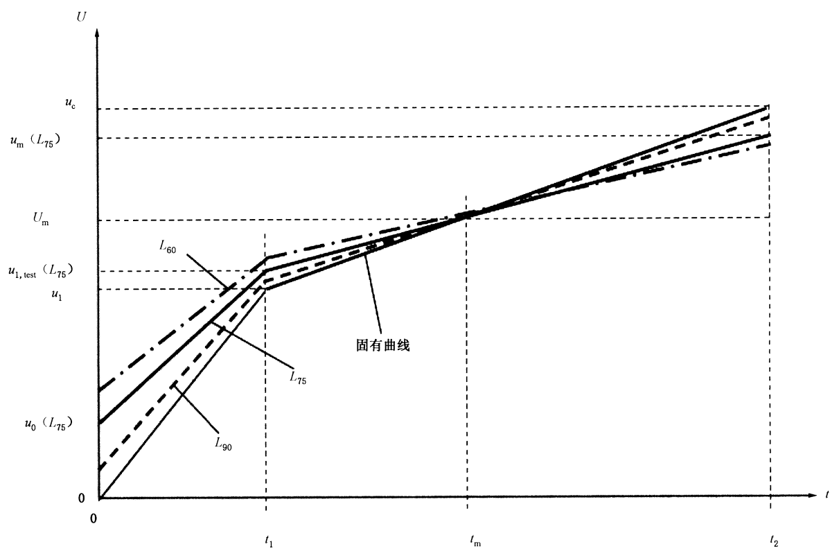
图 A.3 L_{90} 、 L_{75} 和 L_{60} 近区故障时, 电源侧 TRV 的实际曲线
