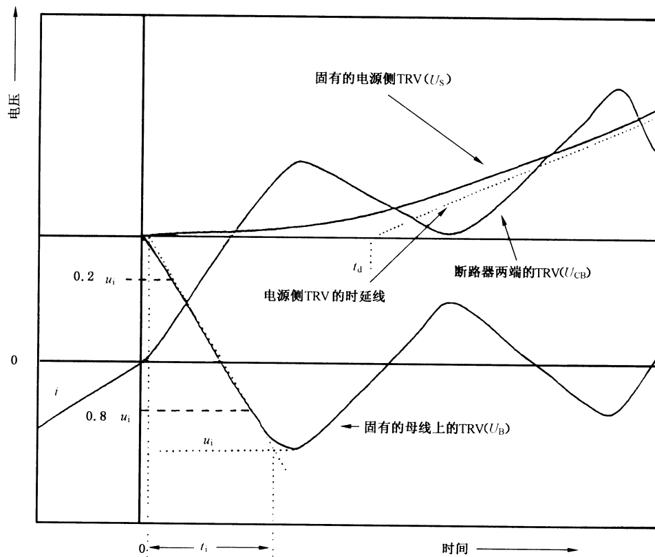
图 12 ITRV 回路以及 ITRV 与 TRV 关系的表示
