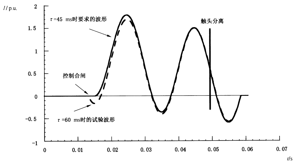
小半波后电流零点时开断
