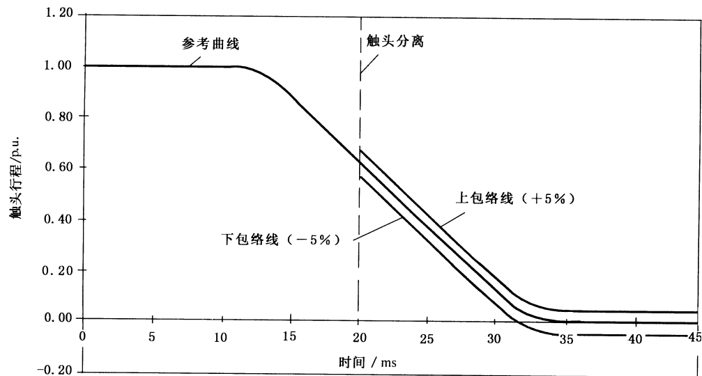
a) 参考的机械行程特性(理想曲线)
