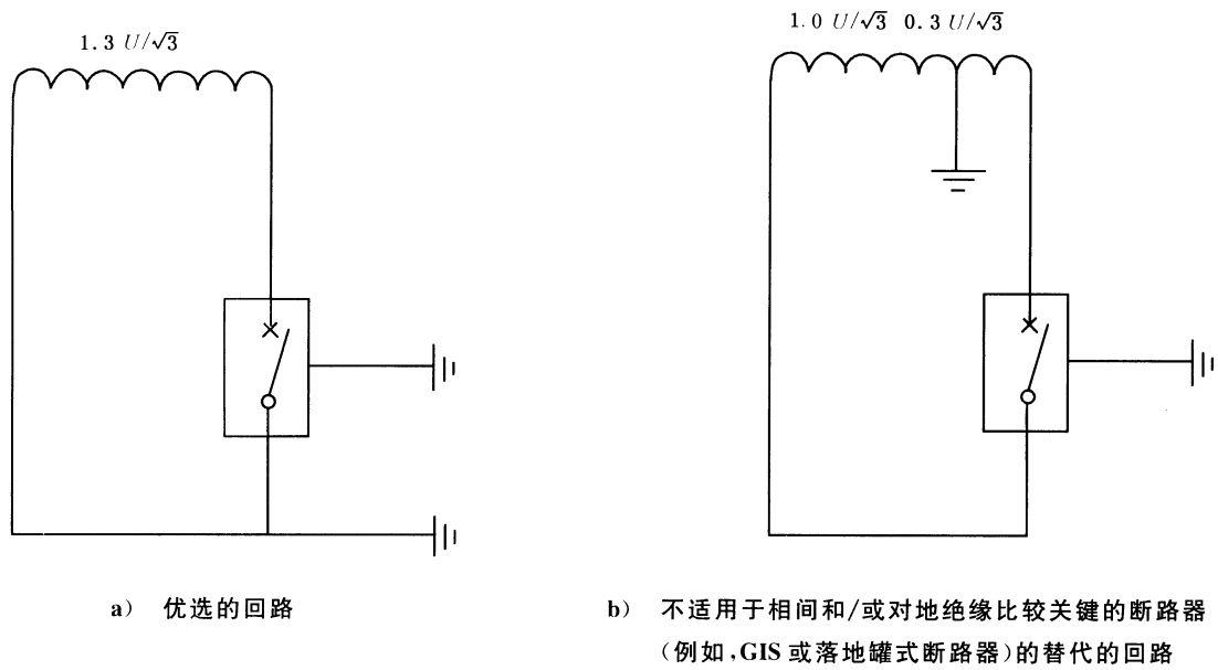
图 28 单相短路试验的试验回路的接地, 首开极系数为 1.3
