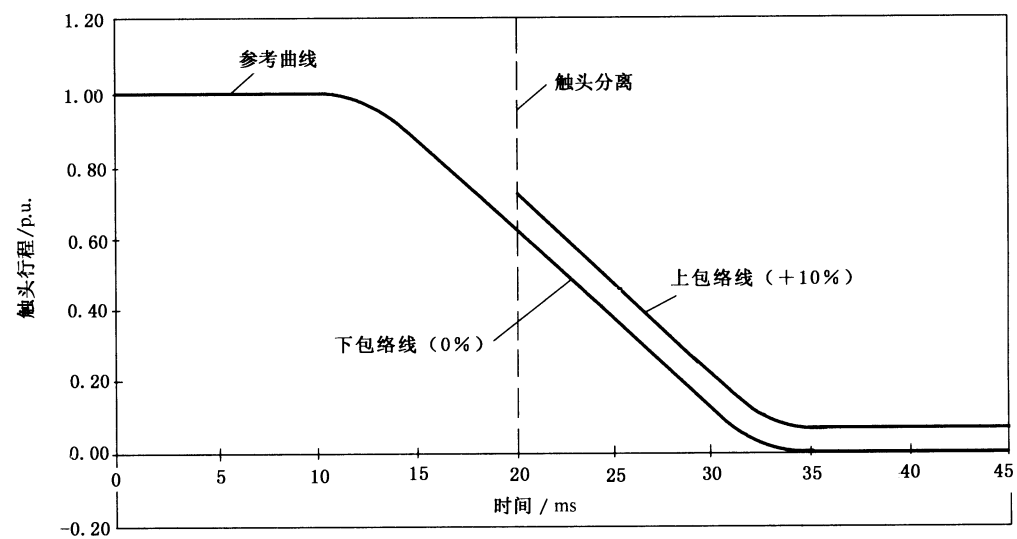
c) 具有以参考曲线为基准完全上移的规定的包络线(+10%,0%)的参考机械行程特性(理想曲线), 本例中触头分离时刻为 t = 20\text{ ms}
