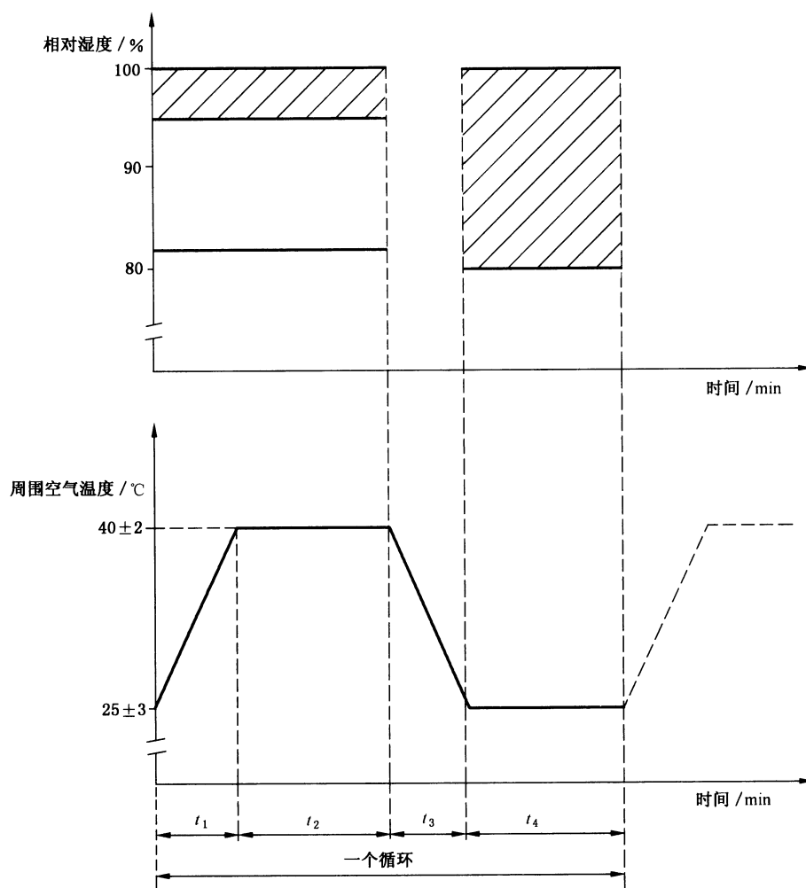
图 18 湿度试验
