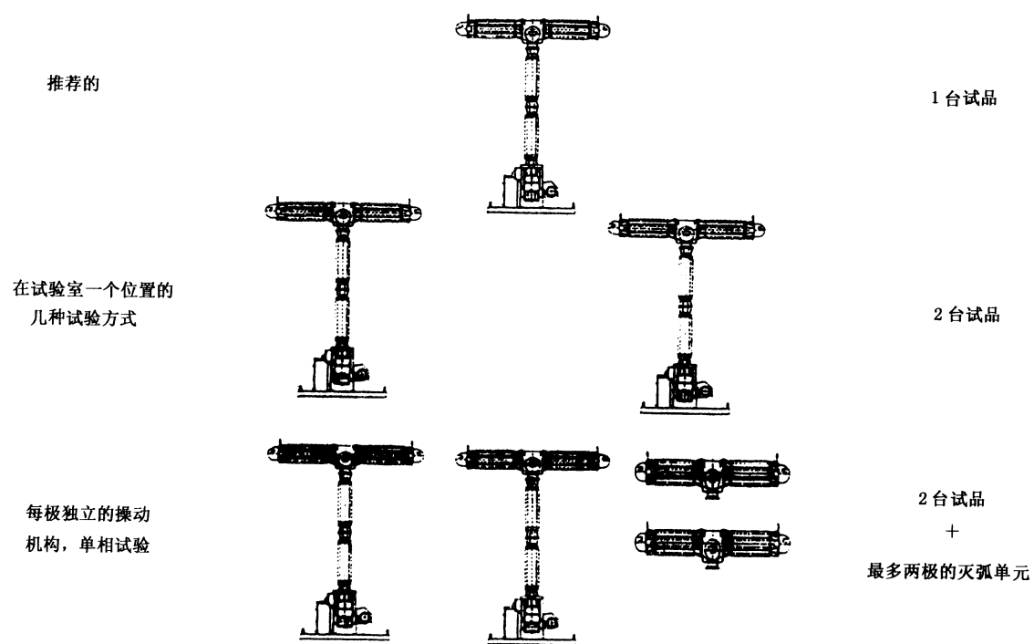
图 21 关合、开断和开合试验允许的试品数量,6.102 中的规定的图示
