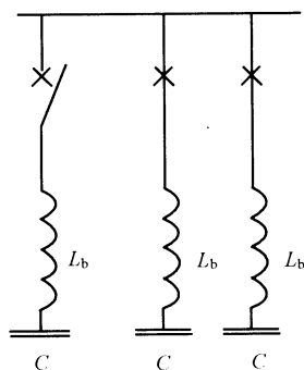
图 H.2 例 2 的回路图
