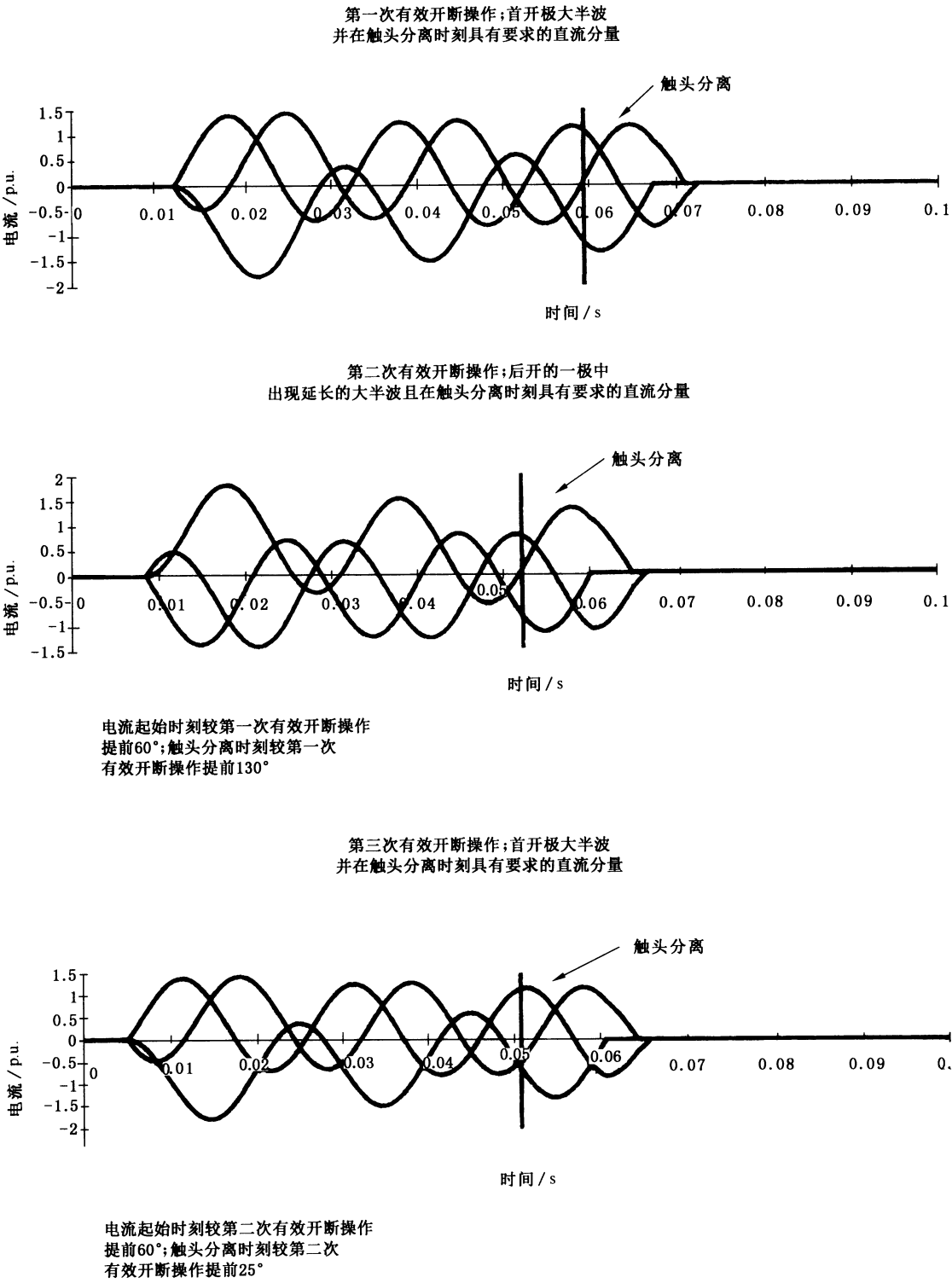
图 31 中性点非有效接地系统中(首开极系数 1.5)三相试验时三次有效非对称开断操作的图形表示
