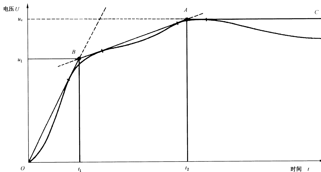
图 E.1 用四参数表示回路的预期瞬态恢复电压——E.2 c) 1) 的情况
