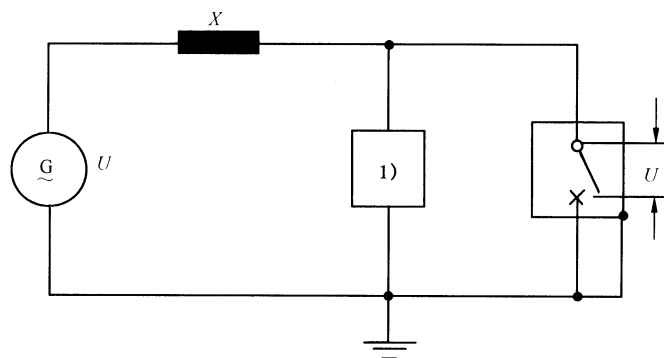
图 52 利用两个相差 120^\circ 的电压进行失步试验的试验回路
