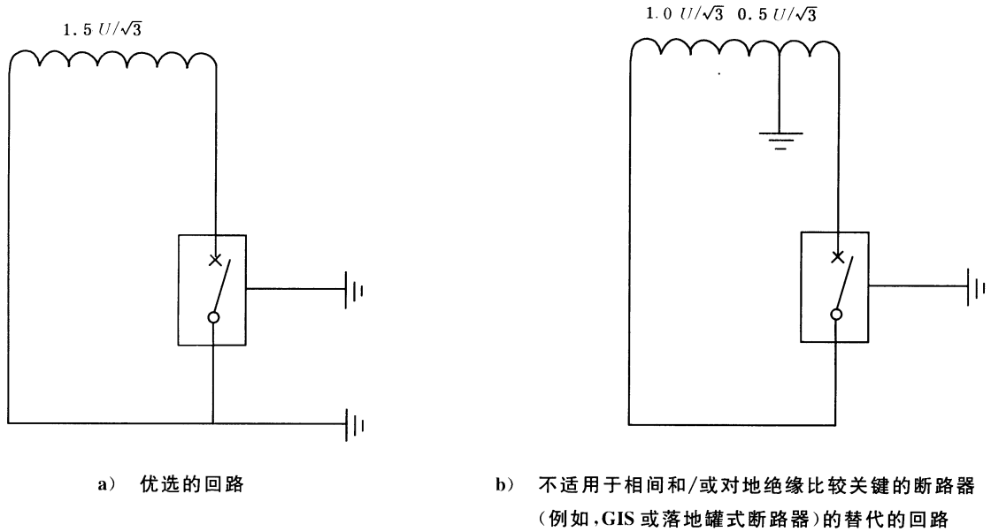
图 27 单相短路试验的试验回路的接地, 首开极系数为 1.5
