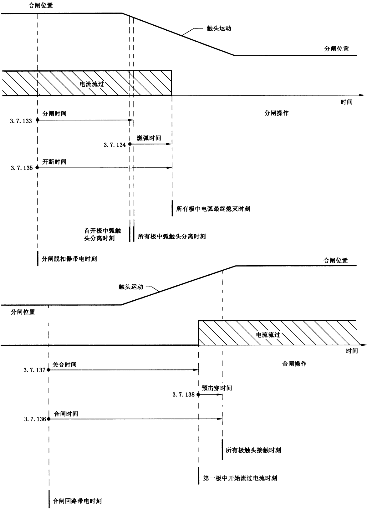
图 2 没有开合电阻的断路器的分闸和合闸操作
